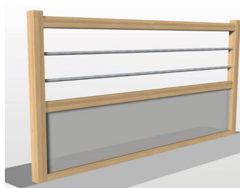
2 tubes + soubassement plexiglass Crystal
